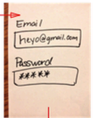
Fig. 1: Welcome
